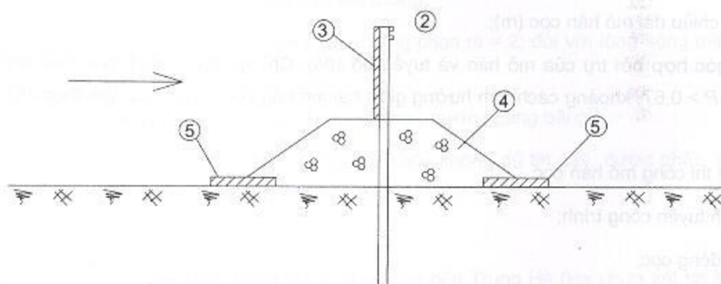
Hình 13 - Kết cấu mô hàn cọc bê tông cốt thép
